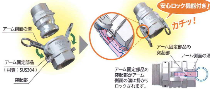
カムロックアルミ構造
