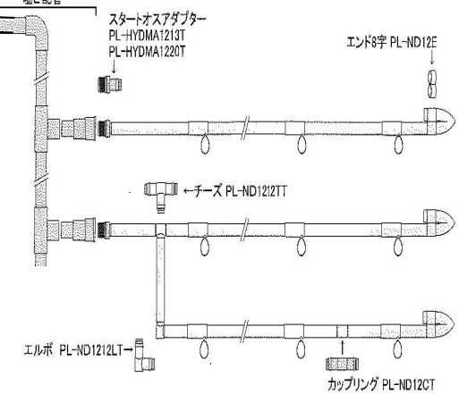
ハイドロ配管
