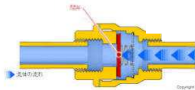
チェックバルブ構造 バキュームブレーカー
