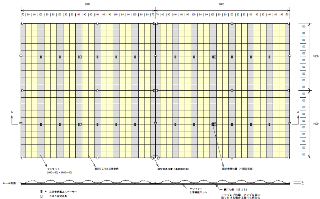
ツタサンオイデパネル敷設図
